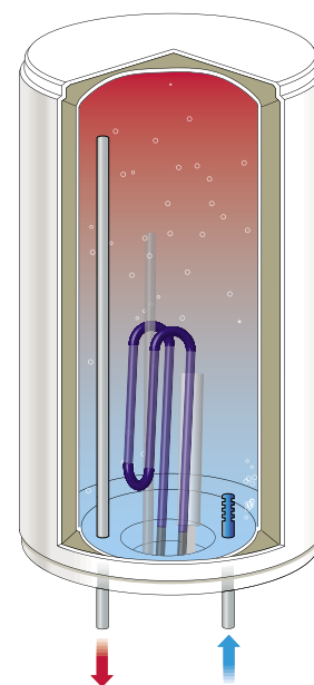
Függőleges telepítés
