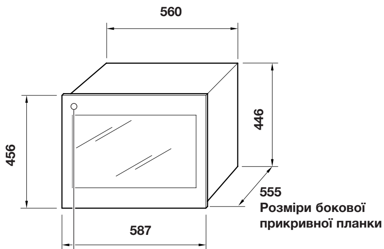
Розміри винної шафи
