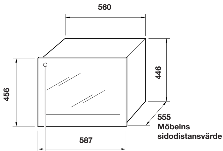
Källarens dimensioner
