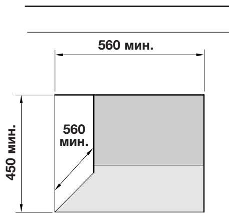
Размери на отделението
