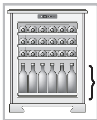
SERVERING 42 flasker (50 % liggende og 50 % stående) 3 stativer brukt
