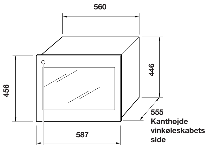
Vinkøleskabets mål
