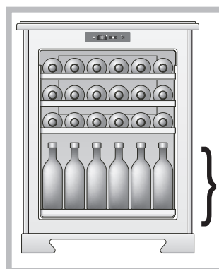
SERVERING 42 flasker (den ene halvdel liggende og den anden halvdel stående) brug af tre riste
