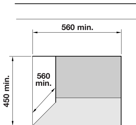
Dimensiunile compartimentului
