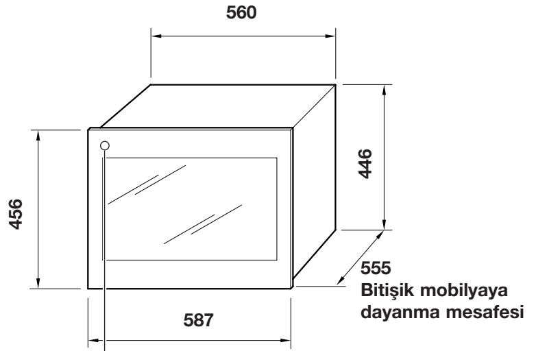
Dolabın boyutları
